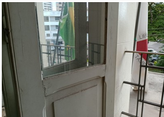
Pará de Minas Fórum Desembargador Pedro Nestor Deterioração contínua da massa no vidro de fechamento das janelas do 1º pavimento. (foto 19) Imagem: Gabriela Conceição – 02/01/2023
