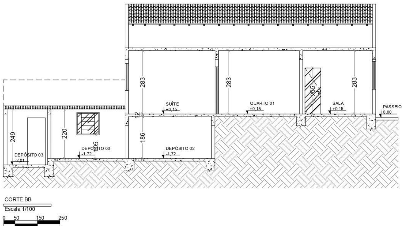
Corte BB – Desenho arquitetônico Karina Morato - CAU-MG A38.403-8 – Janeiro de 2026 - Arquivo Prefeitura de Pará de Minas
