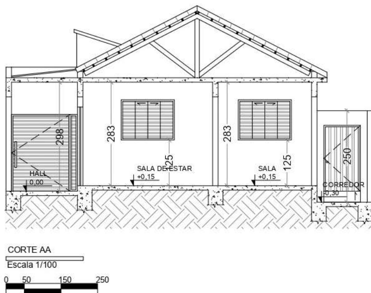
Corte AA – Desenho arquitetônico Karina Morato - CAU-MG A38.403-8 – Janeiro de 2026 - Arquivo Prefeitura de Pará de Minas
