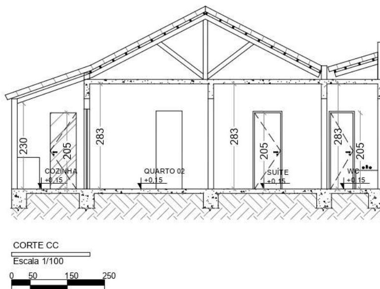
Corte CC – Desenho arquitetônico Karina Morato - CAU-MG A38.403-8 – Janeiro de 2026 - Arquivo Prefeitura de Pará de Minas
