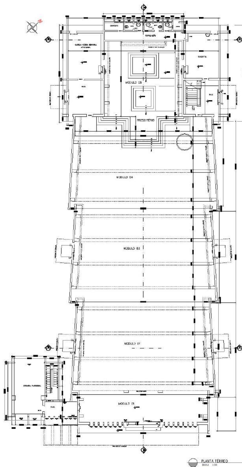
Planta Térreo – Desenho arquitetônico Karina Morato - CAU-MG A38.403-8 – Dezembro de 2022 Arquivo Prefeitura de Pará de Minas
